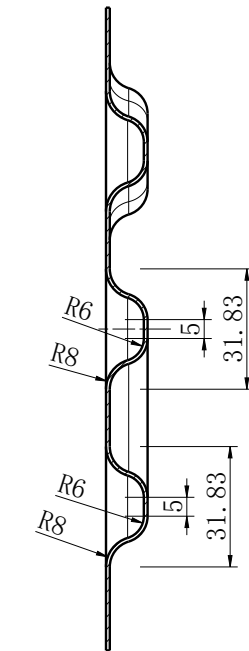
截面 A-A
