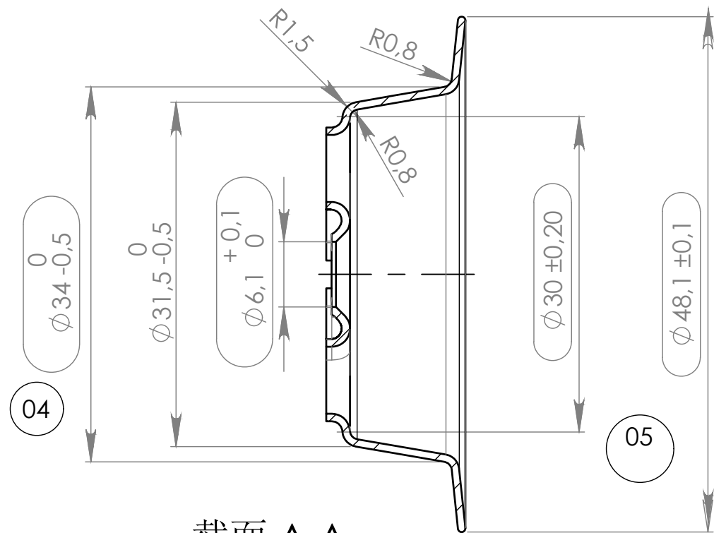
截面 A-A 比例 2:1
